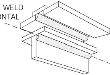
(D) OVERHEAD POSITION 4F
