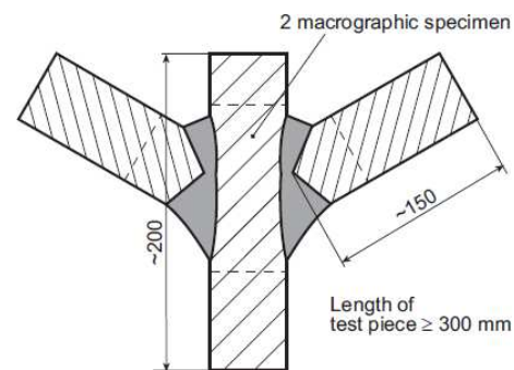
Fig. 14.3 Y test piece
